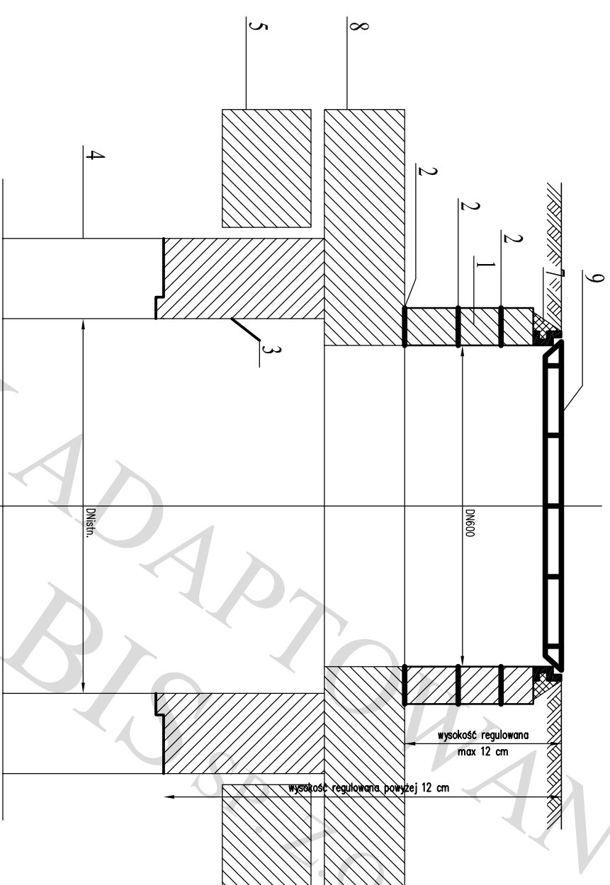
STUDNIA - TYP CIĘŻKI
