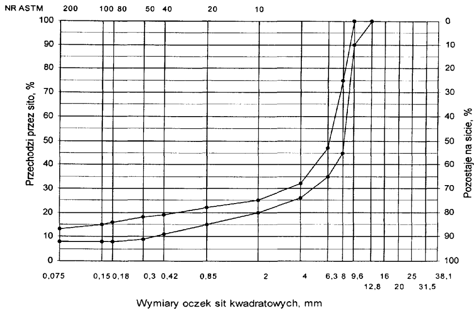
Rys. 6. Krzywe graniczne uziarnienia mieszanki mineralnej SMA od 0 do 9,6 mm do warstwy ściernalnej nawierzchni drogi o obciążeniu ruchem od KR3 do KR6
